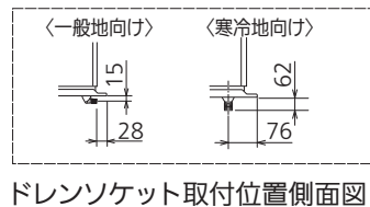
ドレンソケット取付位置側面図
