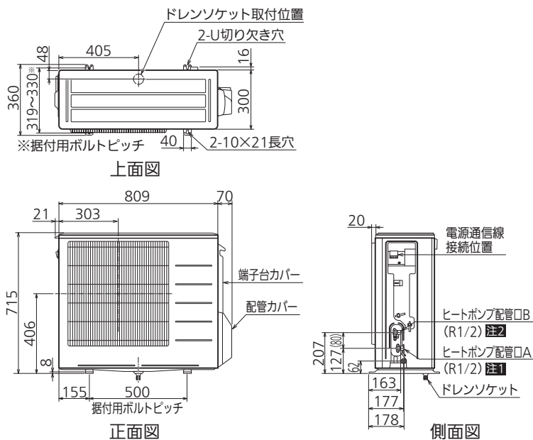
ドレンソケット取付位置側面図
