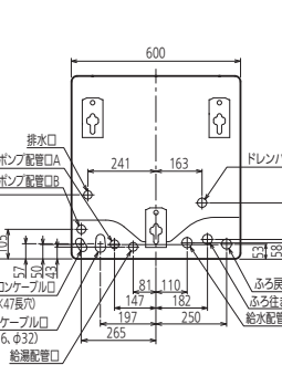
配管位置上面透視図
