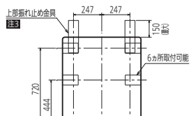
上面図(Dタイプ)
