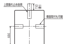
上面図(Dタイプ以外)
