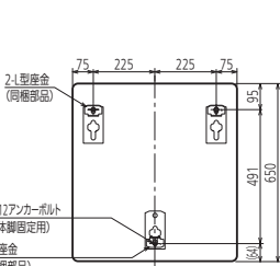
アンカーボルト位置上面透視図 (標準施工時)
