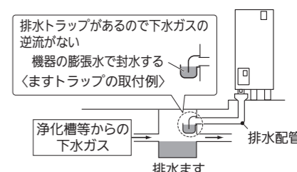
〈図2〉排水口と排水ホッパーの中心を合わせる
