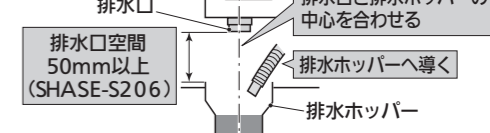
〈図3〉排水ホースの正しい取り付け方
