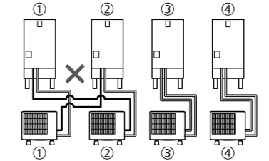
4台連結の場合におけるシステム①と②で配管誤接続例
