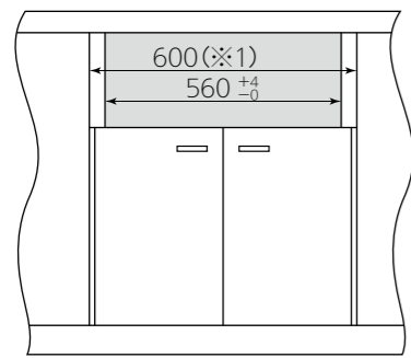
正面図
