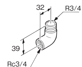
⑦特殊エルボ GT-54F
