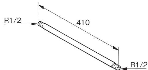
⑧ステンレスニップル
