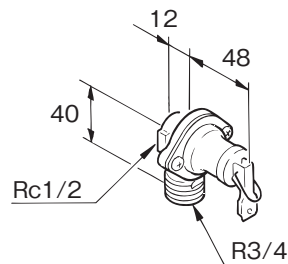
②逃し弁(保温筒付)GT-T19F
