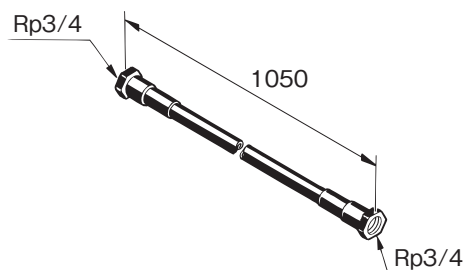
④絶縁パイプ GT-60F
