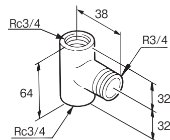
③逃し弁特殊チーズ GT-55F
