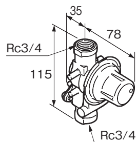
①減圧弁(保温筒付)GT-T8F
