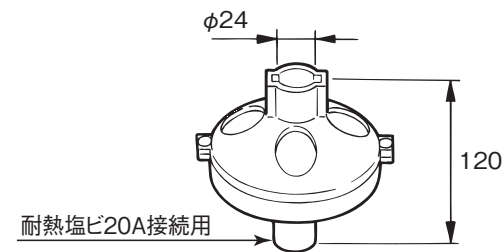
⑥ホッパー(上・下) GT-70G
