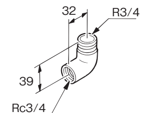
⑦特殊エルボ GT-54G
