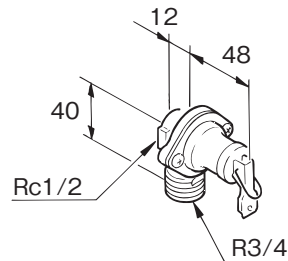
②逃し弁(保温筒付) GT-T19G
