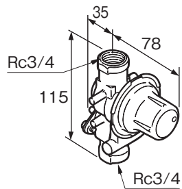
①減圧弁(保温筒付) GT-T8G
