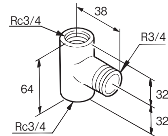
③逃し弁特殊チーズ GT-55G
