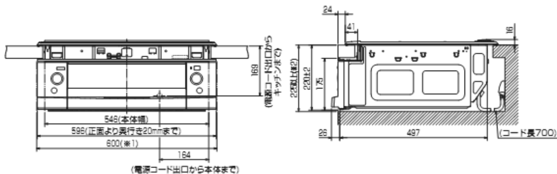
正面図
