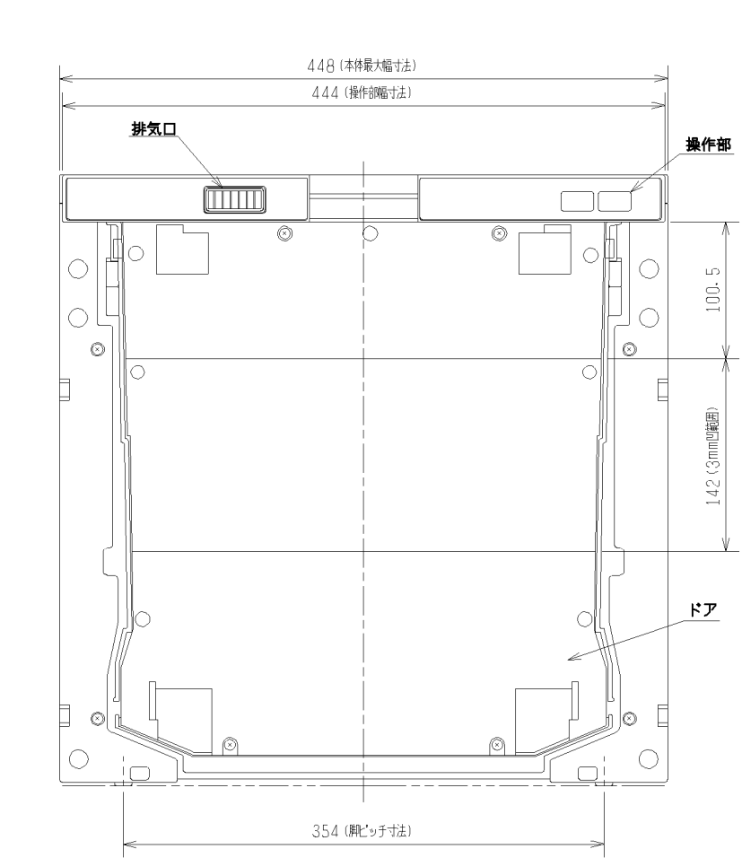
【正面図】
