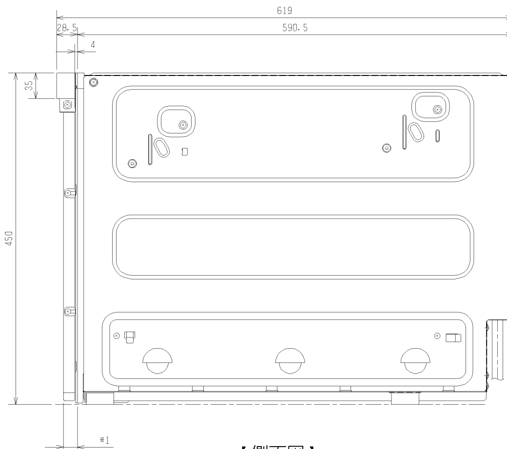
【側面図】
