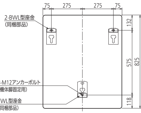
アンカーボルト位置上面透視図 (標準施工)
