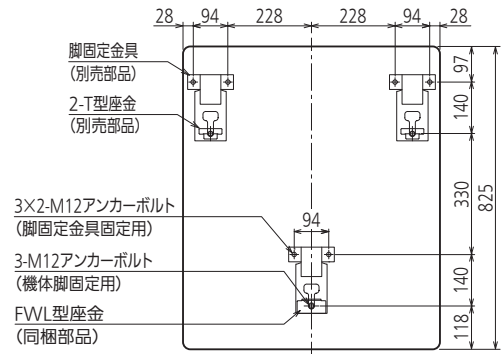
アンカーボルト位置上面透視図 (標準施工できない場合)
