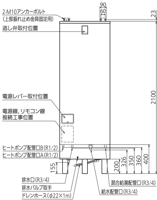
正面図
