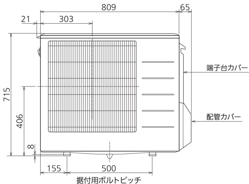
正面図
