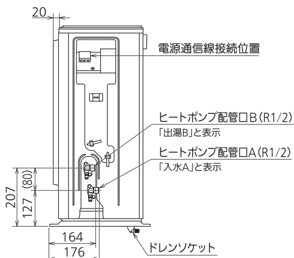
側面図
