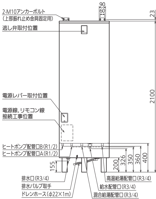
正面図
