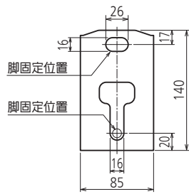
機体脚詳細図
