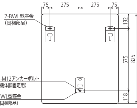
アンカーボルト位置上面透視図 (標準施工)
