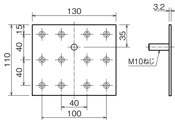
〈脚固定金具寸法図(単位:mm)〉
