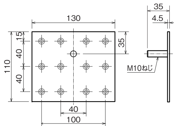
〈脚固定金具寸法図(単位:mm)〉
