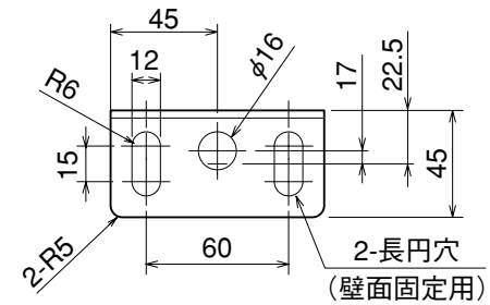
〈部品寸法図(単位:mm)〉
