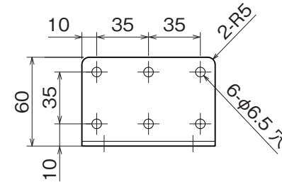
〈部品寸法図(単位:mm)〉
