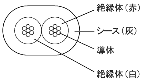
構造図
