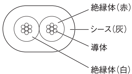
構造図
