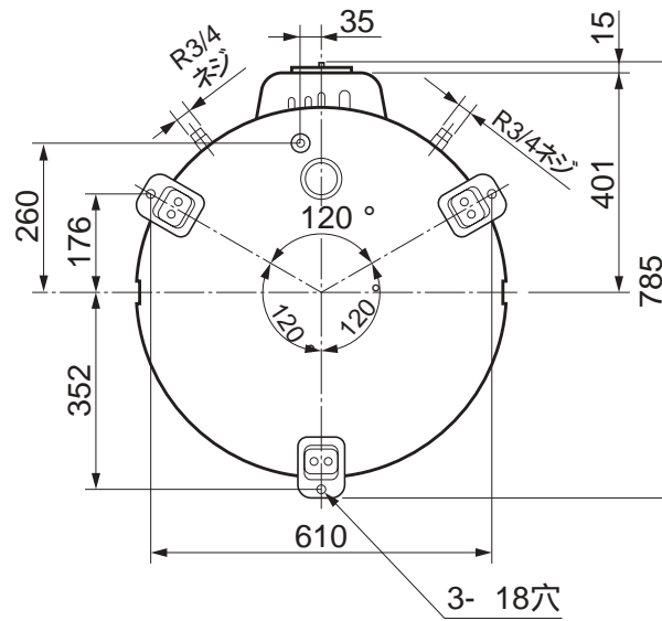
底面図
