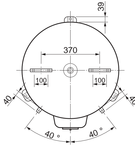
上面図
