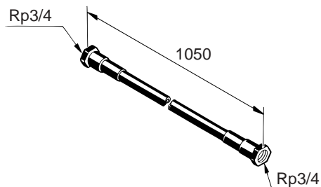
絶縁パイプ GT-60D
