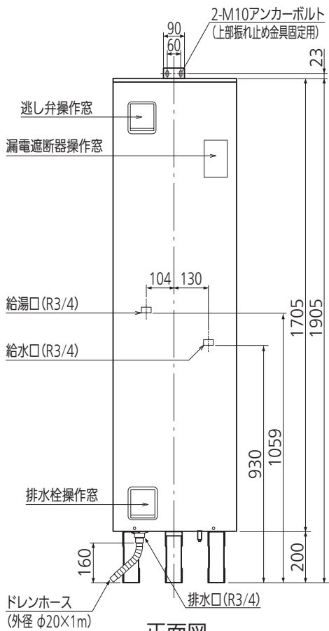
正面図
