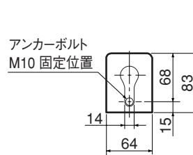
器体脚詳細図
