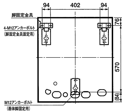
脚固定金具使用時:上面透視図 [SRT-3767CFD-BL、SRT-4667CFD-BL]
