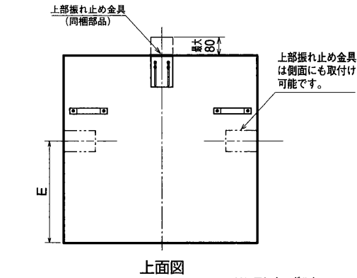
上面図
