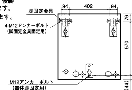
脚固定金具使用時(上面透視図) [SRT-3765U-BL、SRT-4665U-BL]
