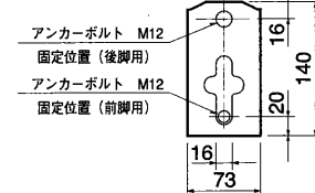
配管、アンカーボルト位置：上面透視図 [SRT-5565U-BL]
