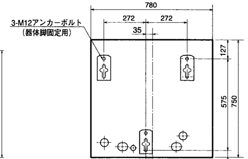
アンカーボルト位置(上面透視図) [SRT-5565U-BL]
