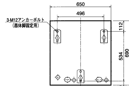
アンカーボルト位置(上面透視図) [SRT-3765U-BL、SRT-4665U-BL]
