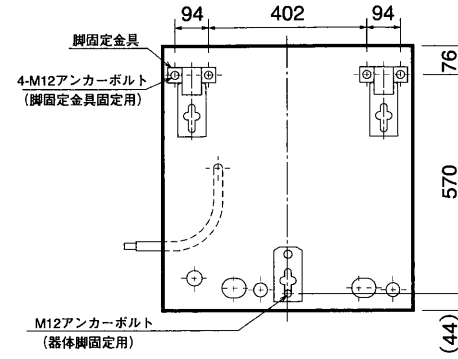
脚固定金具使用時：上面透視図 [SRT-3765U-BL, SRT-4665U-BL]
