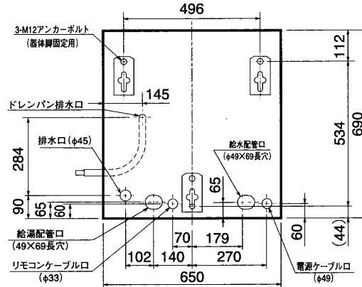
配管、アンカーボルト位置：上面透視図 [SRT-3765U-BL, SRT-4665U-BL]
