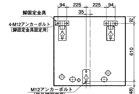
脚固定金具使用時(上面透視図) [SRT-5565U-BL]
