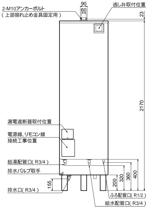
正面図
