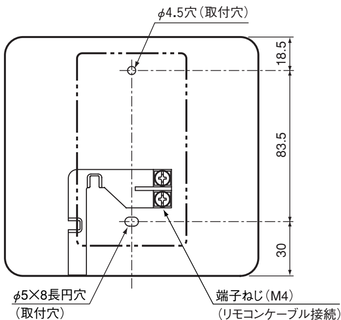
背面図
