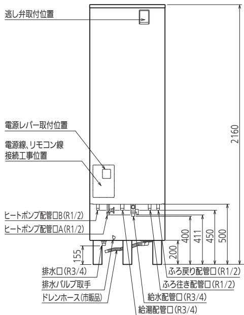
正面図
