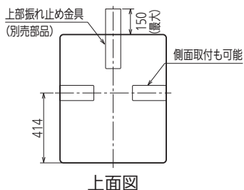
上面図
