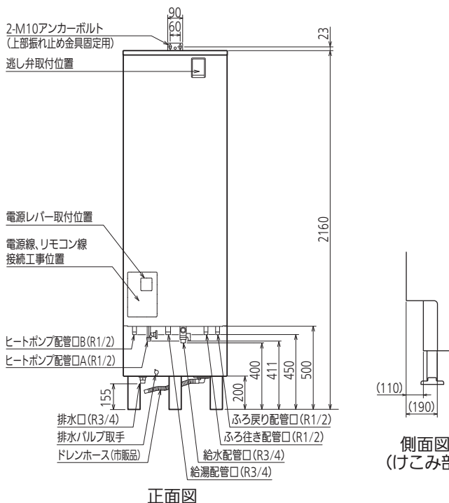
正面図
