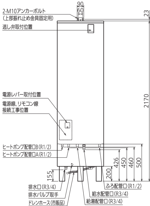
正面図
