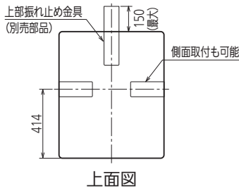
上面図
