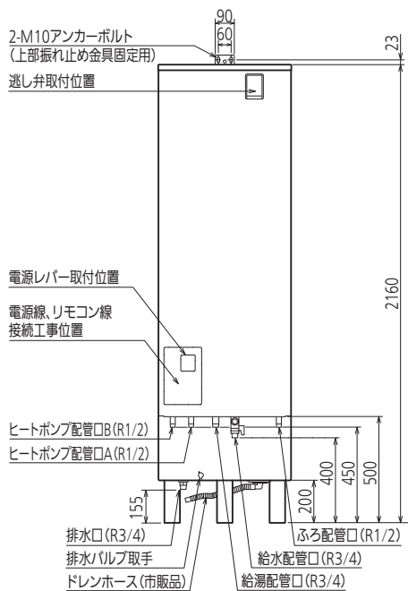
正面図
