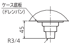
排水口寸法
