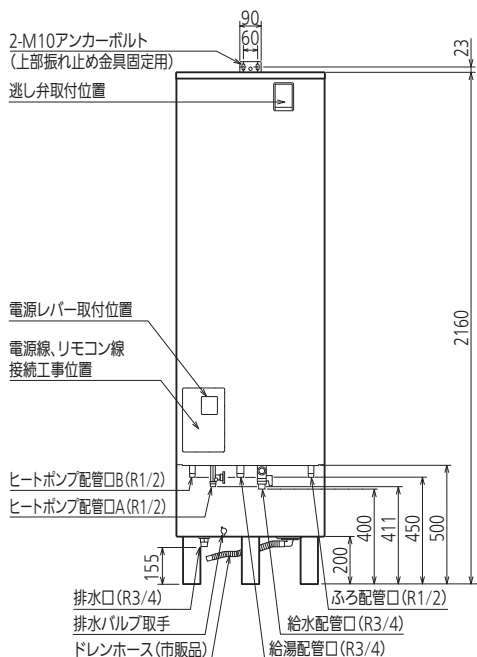
正面図
