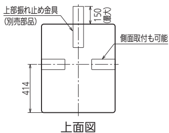
上面図
