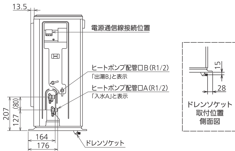
右側面図 (配管カバーを外した図)
