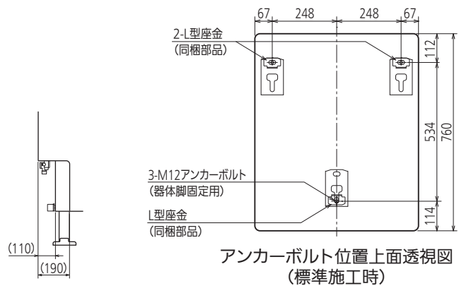
側面図 (けこみ部)
