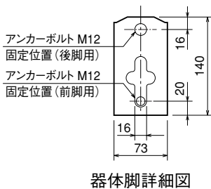
器体脚詳細図
