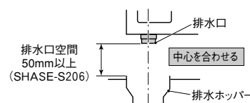
〈図2〉排水口付近拡大図
