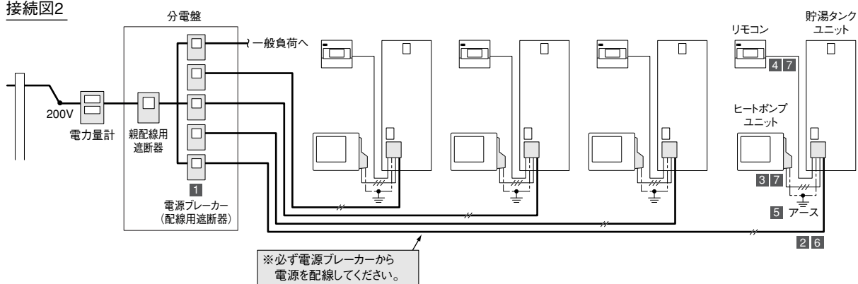
接続図2
