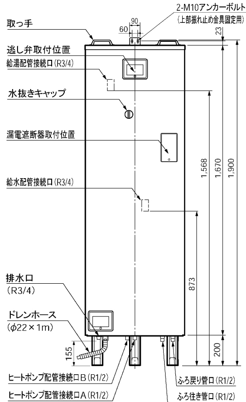
正面図
