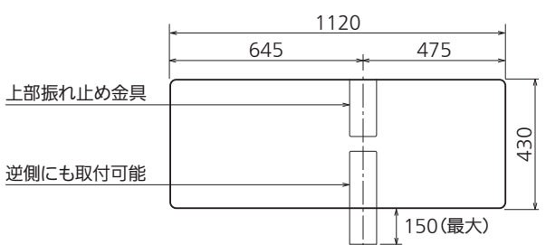
上面図
