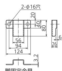
脚固定金具
