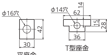
平座金
