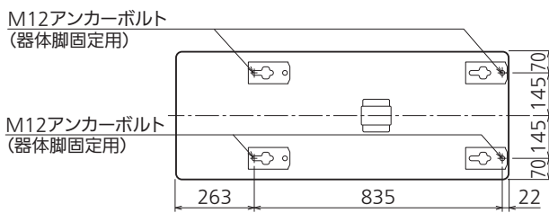
アンカーボルト位置上面透視図
