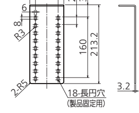
18-長円穴 (製品固定用)
