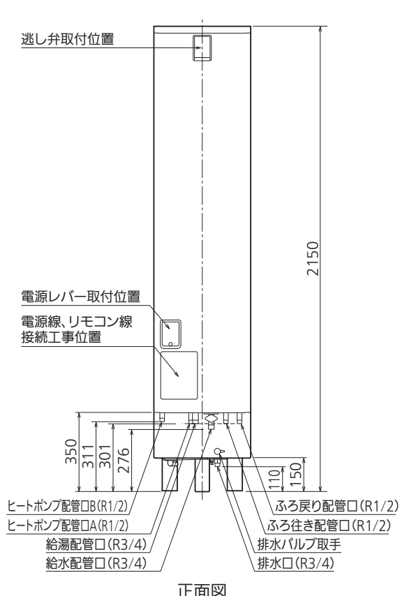
正面図
