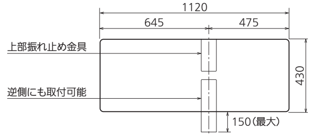
上面図
