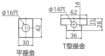
平座金
