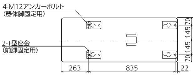
アンカーボルト位置上面透視図
