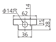
T型座金 (同梱部品)
