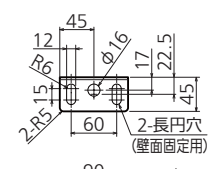
2-長円穴 (壁面固定用)
