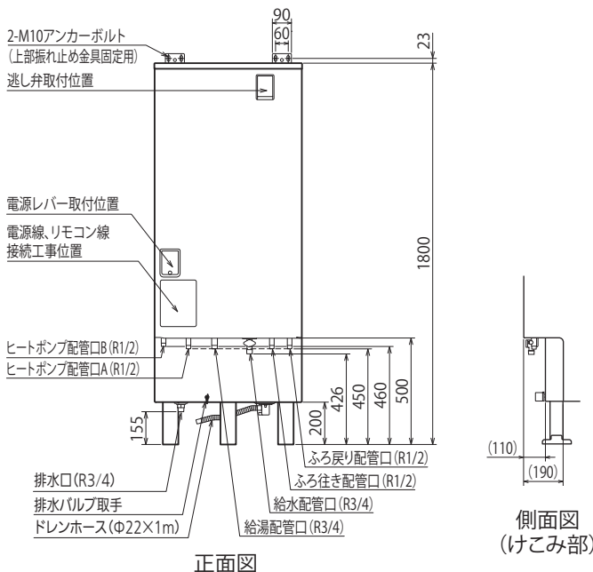
正面図
