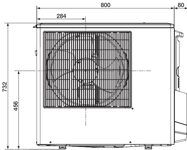
正面図
