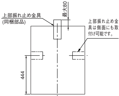
上面図
