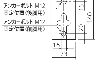
器体脚詳細図
