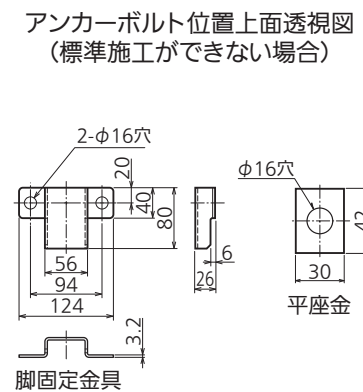
脚固定金具(別売部品)
