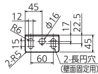
排水口寸法
