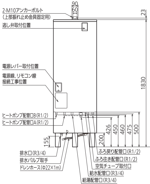
正面図
