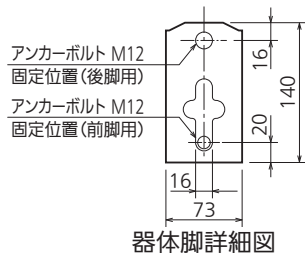
器体脚詳細図
