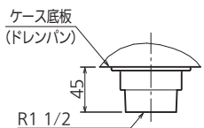
排水口寸法
