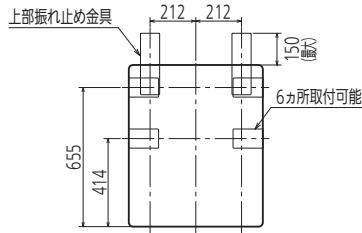
上面図
